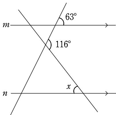
図1 m \parallel n
