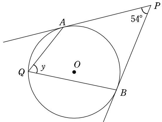
図2 直線 PA , PB は円 O の接線
